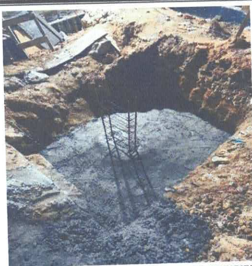
FOTO 15: CONCRETO SIMPLES USINADO FCK=35MPA, BOMBEADO, LANÇADO E ADENSADO NA INFRAESTRUTURA.
