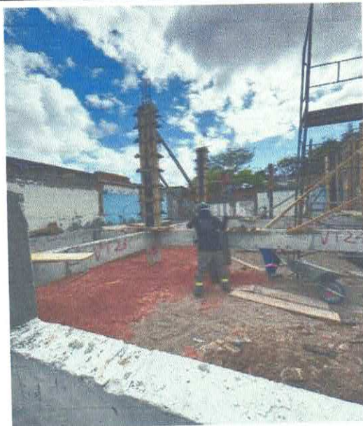
FOTO 06: ATERRO MANUAL DE VALAS COM AREIA PARA ATERRO E COMPACTAÇÃO MECANIZADA.
