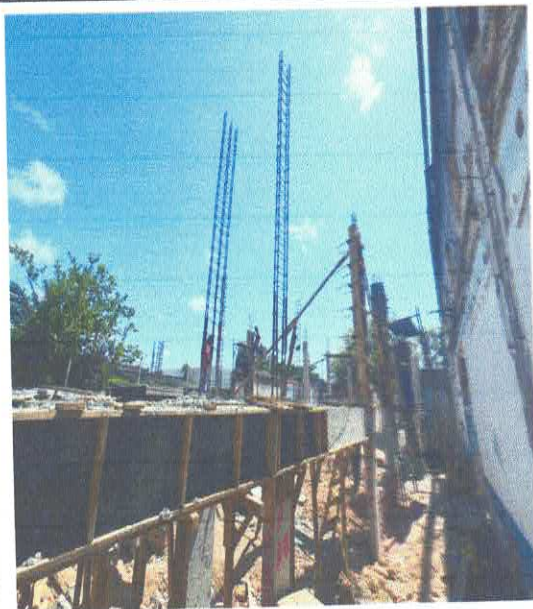
FOTO 22: ARMAÇÃO DE PILAR OU VIGA DE ESTRUTURA CONVENCIONAL DE CONCRETO ARMADO UTILIZANDO AÇO CA-50 DE 8,0 MM.
